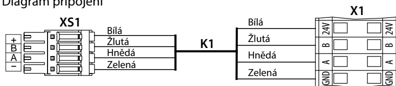
Diagram připojení
